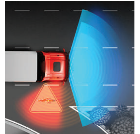
BLIS - SISTEMA INFORMATIVO PUNTI CIECHI Utilizza sensori radar per rilevare pedoni, ciclisti o veicoli nei punti ciechi; avvisa il conducente con segnali visivi e acustici.
